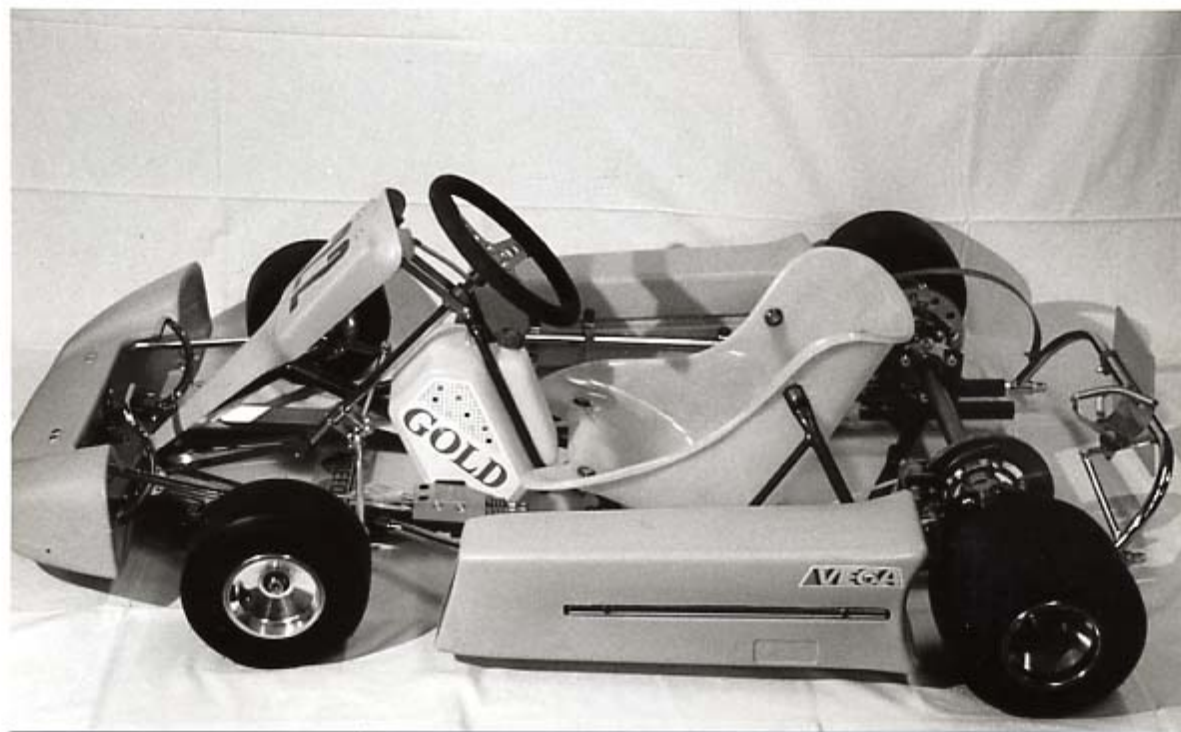
Photo du châssis avec pneumatique
